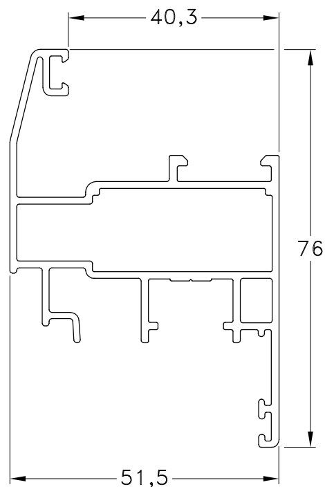
1060891 - Hoja C-16 Peso: 1,08 Kg/m. Largo Std.: 6.150 mm.
