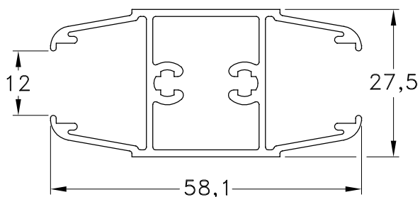
1060730 - Travesaño Hoja 1060787 Peso: 0,80 Kg/m. Largo Std.: 6.030 mm.
