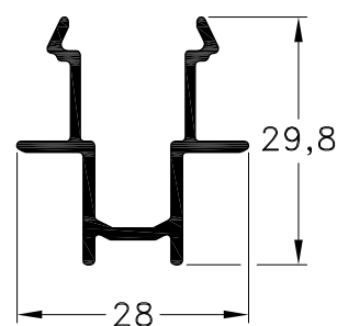
1060569 - Encuentro Cuatro Hojas M-Tres y M-Cinco Peso: 0,33 Kg/m. Largo Std.: 6.030 mm.
