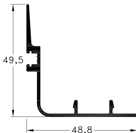
1060556 - Encuentro Peso: 0,44 Kg/m. Largo Std.: 6.030 mm.
