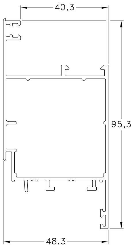
1060848 - Cabezal y Parante Peso: 1,10 Kg/m. Largo Std.: 6.150 mm.
