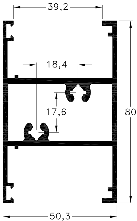
1060544 - Travesaño Peso: 1,71 Kg/m. Largo Std.: 6.030 mm.
