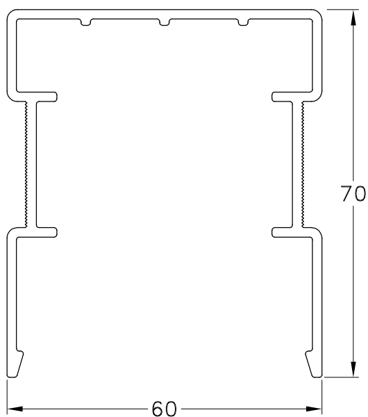
1060599 - Tapa Inercial Peso: 1,15 Kg/m. Largo Std.: 6.030 mm.
