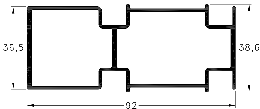
1060856 - Acople Recto Reforzado Peso: 1,27 Kg/m. Largo Std.: 6.030 mm.
