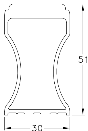
1060518 - Refuerzo Parantes M-Uno, M-Tres y M-Cinco Peso: 1,00 Kg/m. Largo Std.: 6.030 mm.
