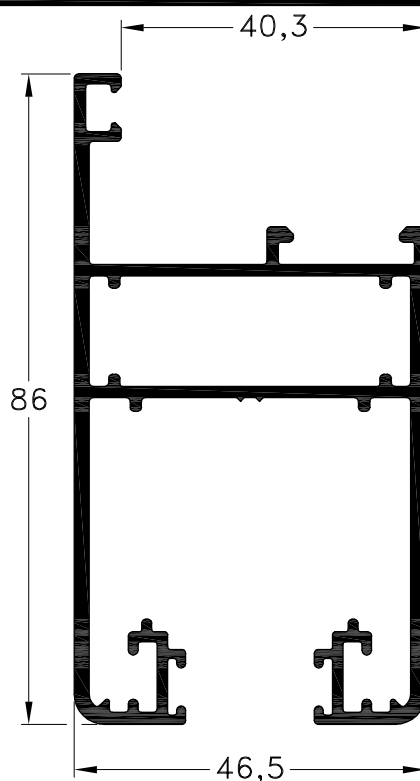
1060580 - Hoja Perimetral con Contravidrio Peso: 1,54 Kg/m. Largo Std.: 6.030 mm.
