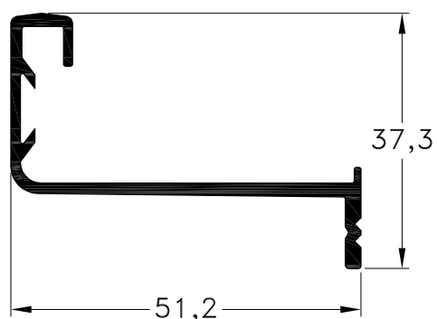
1060558 - Guía Mosquitero Peso: 0,49 Kg/m. Largo Std.: 6.030 mm.
