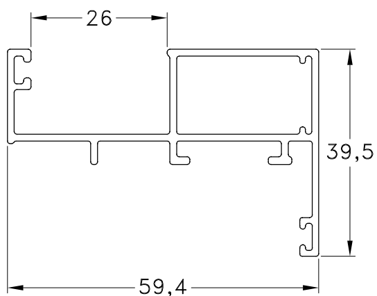
1060774 - Hoja Peso: 0,69 Kg/m. Largo Std.: 6.030 mm.
