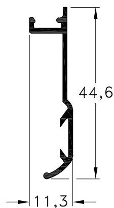
1060862 - Contramarco Peso: 0,21 Kg/m. Largo Std.: 6.150 mm.
