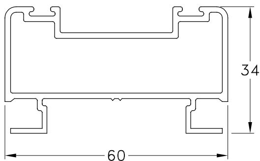
1060597 - Marco Puerta Vaivén Peso: 0,89 Kg/m. Largo Std.: 6.150 mm.
