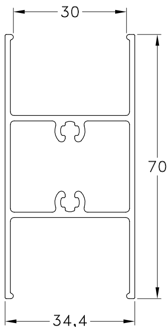
1060172 - Travesaño Peso: 0,90 Kg/m. Largo Std.: 6.030 mm.
