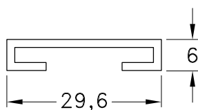
1060566 - Guía de Cierre Puerta Vaivén Peso: 0,21 Kg/m. Largo Std.: 6.030 mm.
