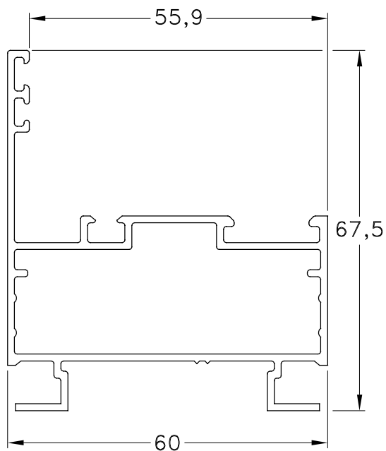
1060779 - Marco Peso: 1,00 Kg/m. Largo Std.: 6.030 mm.
