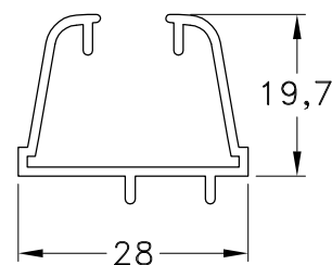
1060749 - Perimetral V.R. Peso: 0,27 Kg/m. Largo Std.: 6.030 mm.
