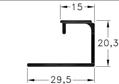
1060559 - Contravidrio 16 mm. para Perfil 1060555 Peso: 0,24 Kg/m. Largo Std.: 6.030 mm.
