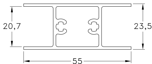
1060681 - Travesaño Hoja 1060742 Peso: 0,70 Kg/m. Largo Std.: 6.030 mm.
