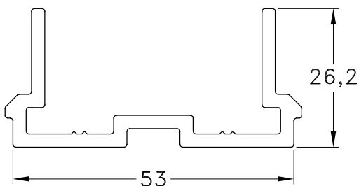
1060600 - Base Inercial Peso: 0,80 Kg/m. Largo Std.: 6.030 mm.
