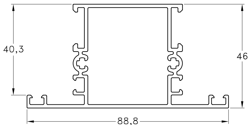
1060888 - Travesaño Ancho Peso: 1,21 Kg/m. Largo Std.: 6.030 mm.
