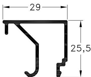
1060876 - Contravidrio Peso: 0,33 Kg/m. Largo Std.: 6.030 mm.
