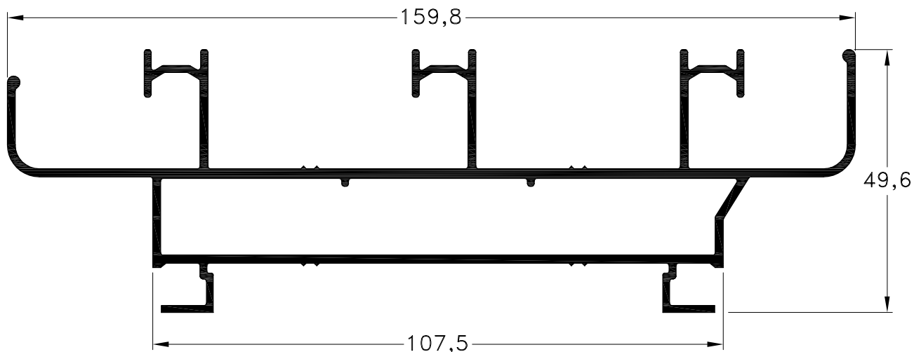
1060873 - Marco Perimetral de Tres Guías Peso: 2,10 Kg/m. Largo Std.: 6.030 mm.
