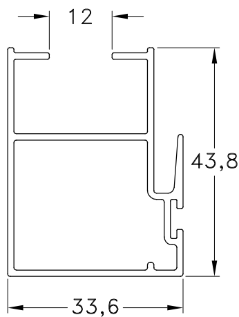
1060822 - Parante Central V.S. Peso: 0,60 Kg/m. Largo Std.: 6.150 mm.
