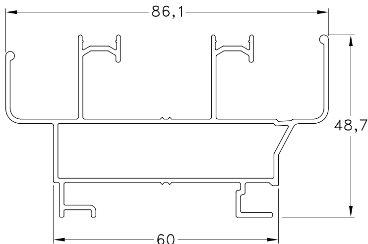
1060802 - Marco Perimetral Peso: 1,09 Kg/m. Largo Std.: 6.030 mm.
