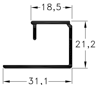
1060173 - Contravidrio de 12 mm. V.S. Peso: 0,26 Kg/m. Largo Std.: 6.030 mm.
