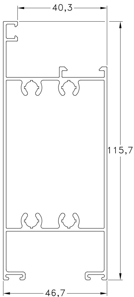
1060849 - Zócalo Peso: 1,54 Kg/m. Largo Std.: 6.030 mm.
