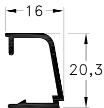
1060523 - Contravidrio Peso: 0,17 Kg/m. Largo Std.: 6.030 mm.
