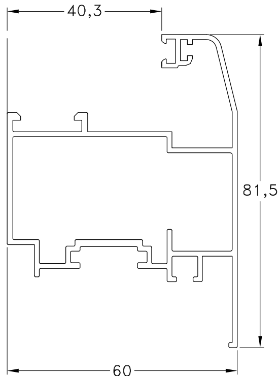
1060786 - Hoja Ventana Desplazable Peso: 1,18 Kg/m. Largo Std.: 6.150 mm.
