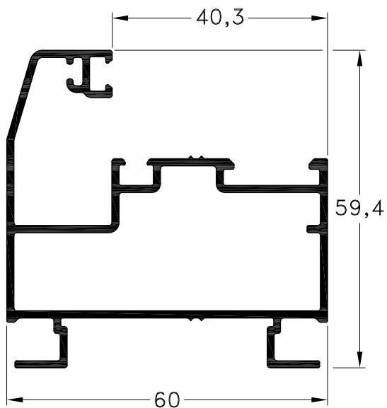
1060895 - Marco No-Coplanar Peso: 1,08 Kg/m. Largo Std.: 6.150 mm.
