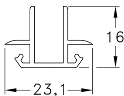
1060590 - Encuentro Cuatro Hojas M-Uno Peso: 0,20 Kg/m. Largo Std.: 6.030 mm.
