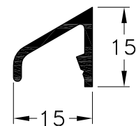
1060200 - Bota-Agua Peso: 0,15 Kg/m. Largo Std.: 6.030 mm.
