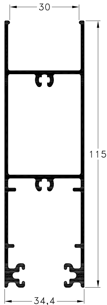
1060167 - Zócalo Alto Peso: 1,47 Kg/m. Largo Std.: 6.030 mm.
