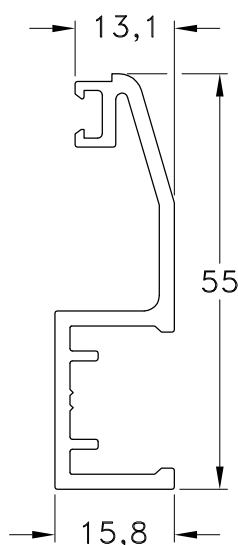
1060859 - Soporte Vidrio Paño Fijo Peso: 0,57 Kg/m. Largo Std.: 6.030 mm.
