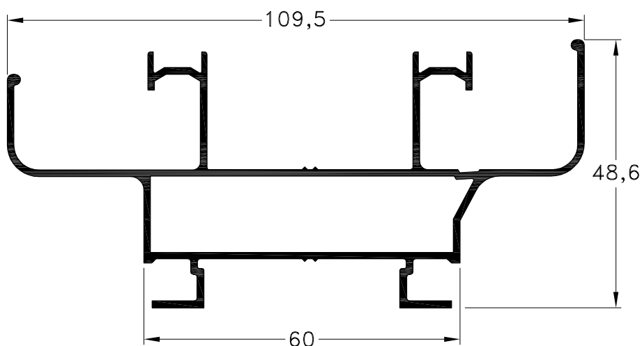
1060729 - Marco Perimetral Peso: 1,20 Kg/m. Largo Std.: 6.030 mm.
