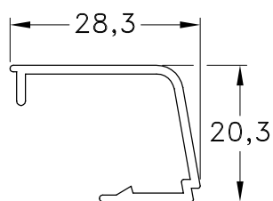
1060380 - Contravidrio Peso: 0,22 Kg/m. Largo Std.: 6.030 mm.
