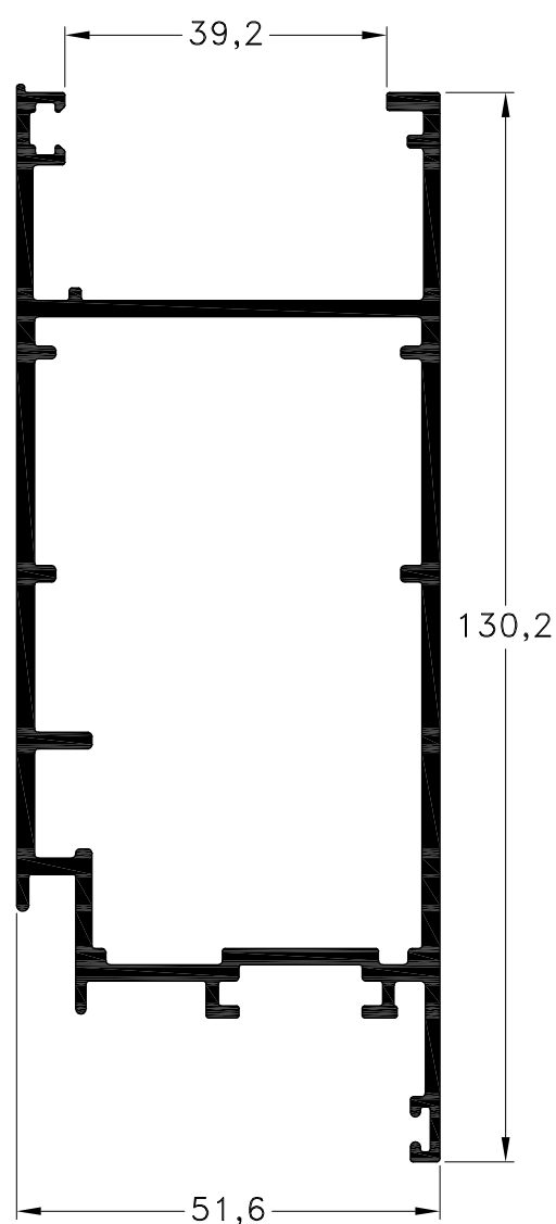
1060500 - Cabezal y Parante Reforzado Peso: 2,17 Kg/m. Largo Std.: 6.150 mm.
