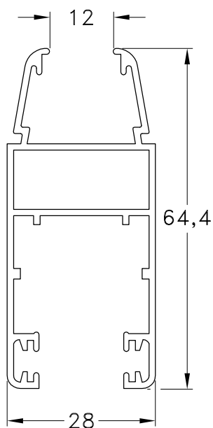
1060787 - Hoja Perimetral V. Laminado Peso: 0,76 Kg/m. Largo Std.: 6.030 mm.
