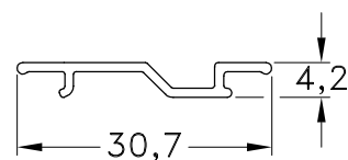
1040129- Tapa Doble Compensador Peso: 0,12 Kg/m. Largo Std.: 6.030 mm.
