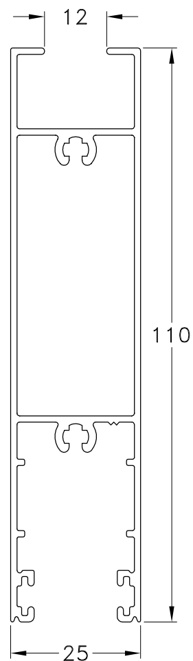
1060824 - Zócalo Alto V.S. Peso: 1,11 Kg/m. Largo Std.: 6.030 mm.
