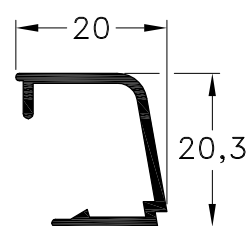
1060525 - Contravidrio Peso: 0,19 Kg/m. Largo Std.: 6.030 mm.
