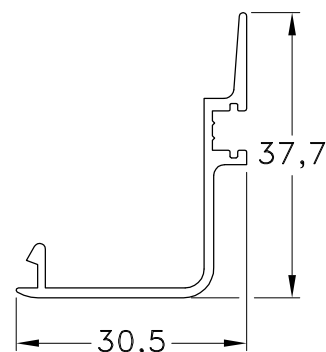
1060743 - Encuentro Central Peso: 0,29 Kg/m. Largo Std.: 6.030 mm.
