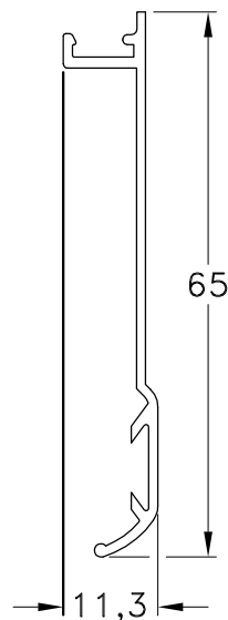
1060857 - Contramarco Peso: 0,27 Kg/m. Largo Std.: 6.150 mm.
