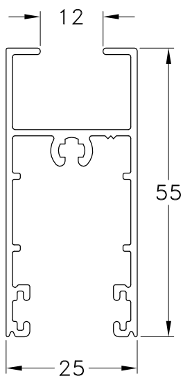
1060820 - Cabezal / Zócalo V.S. Peso: 0,62 Kg/m. Largo Std.: 6.030 mm.
