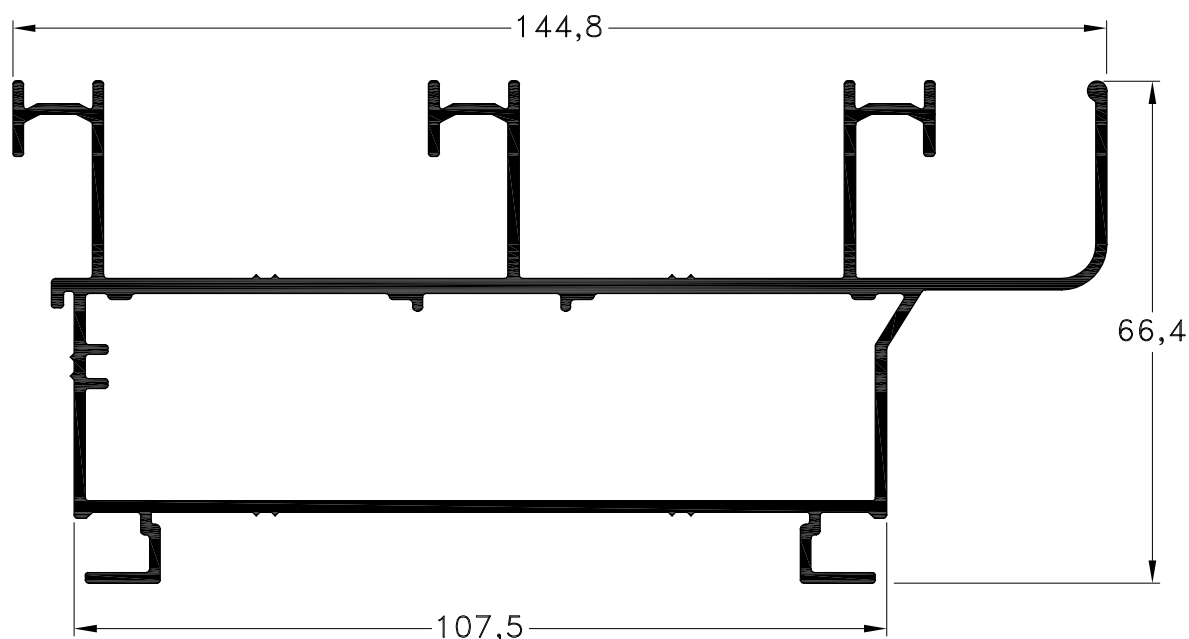
1060874 - Marco Perimetral de Tres Guías Peso: 2,30 Kg/m. Largo Std.: 6.030 mm.
