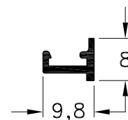
1060310 - Tapa Terminación Coplanar Marco Peso: 0,07 Kg/m. Largo Std.: 6.150 mm.
