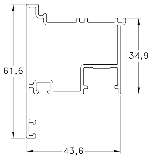
1060892 - Inversor C-16 Peso: 0,82 Kg/m. Largo Std.: 6.150 mm.
