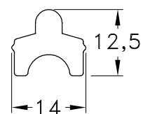
1060608 - Sobre Guía Marco Peso: 0,26 Kg/m. Largo Std.: 6.030 mm.
