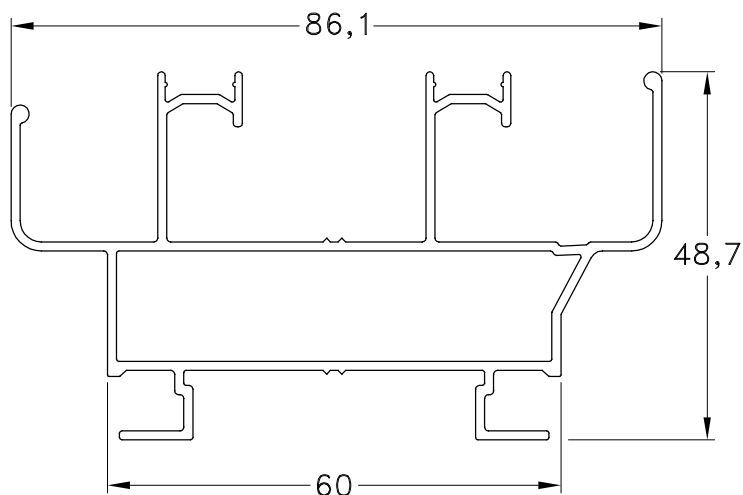
1060803 - Marco Perimetral Peso: 1,09 Kg/m. Largo Std.: 6.030 mm.
