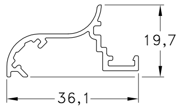
1060727 - Embellecedor de Marco Peso: 0,26 Kg/m. Largo Std.: 6.030 mm.
