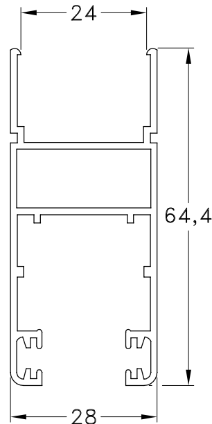
1060742 - Hoja Perimetral D.V.H. Peso: 0,76 Kg/m. Largo Std.: 6.030 mm.
