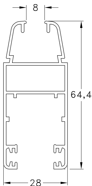
1060741 - Hoja Perimetral V.S. Peso: 0,76 Kg/m. Largo Std.: 6.030 mm.
