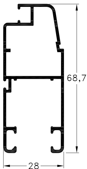
1060560 - Mosquitero Peso: 0,75 Kg/m. Largo Std.: 6.030 mm.
