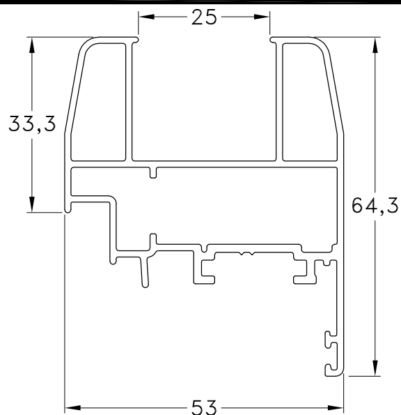
1060826 - Hoja D.V.H. Peso: 1,05 Kg/m. Largo Std.: 6.150 mm.
