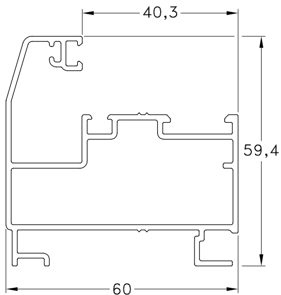
1060893 - Marco No-Coplanar Peso: 1,08 Kg/m. Largo Std.: 6.150 mm.
