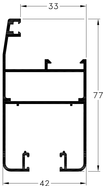
1060712 - Hoja Perimetral con Contravidrio Peso: 1,05 Kg/m. Largo Std.: 6.030 mm.
