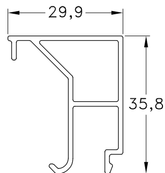
1060773 - Contravidrio P.F. Peso: 0,42 Kg/m. Largo Std.: 6.030 mm.
