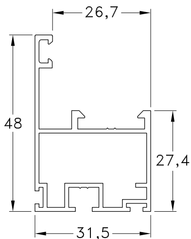
1040507 - Hoja Peso: 0,56 Kg/m. Largo Std.: 6.030 mm.
