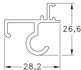
1060843 - Bisagra Tapacinta Peso: 0,34 Kg/m. Largo Std.: 6.150 mm.
