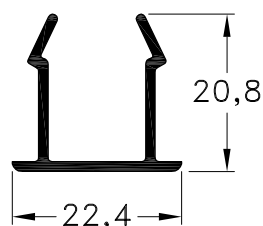
1060573 - Tapa Mosquitero Peso: 0,22 Kg/m. Largo Std.: 6.030 mm.
