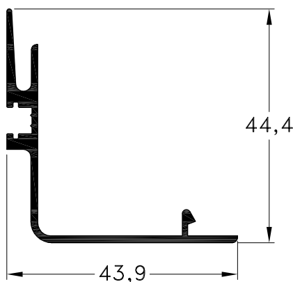
1060713 - Encuentro Peso: 0,40 Kg/m. Largo Std.: 6.030 mm.
