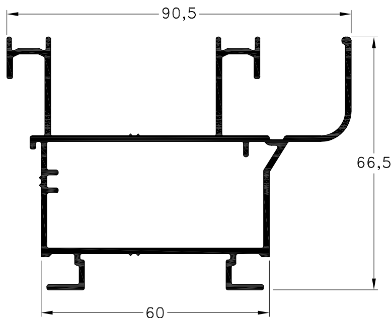
1060554 - Marco Perimetral Peso: 1,48 Kg/m. Largo Std.: 6.030 mm.
