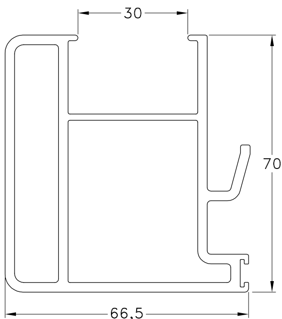
1060170 - Parante Central Reforzado M-Arq. Peso: 2,35 Kg/m. Largo Std.: 6.150 mm.
