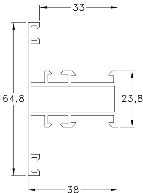
1060733 - Travesaño Hoja con Contravidrio 1060712 Peso: 0,85 Kg/m. Largo Std.: 6.030 mm.
