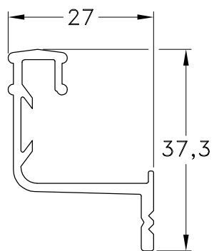
1060574 - Guía Mosquitero Peso: 0,38 Kg/m. Largo Std.: 6.030 mm.
