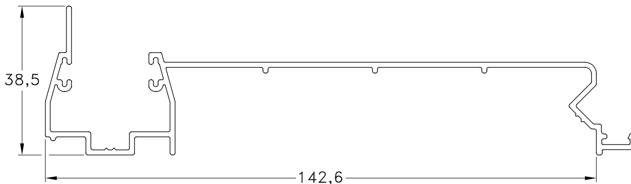
1060579 - Guía Cortina Regulable Peso: 0,99 Kg/m. Largo Std.: 6.150 mm.
