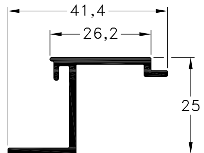
1060545 - Contravidrio de 26 mm. Peso: 0,35 Kg/m. Largo Std.: 6.030 mm.
