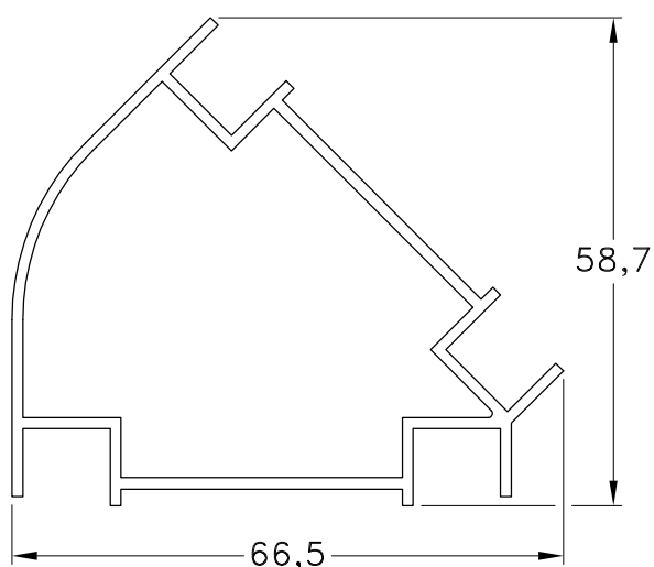
1060563 - Columna Curva a 135°
