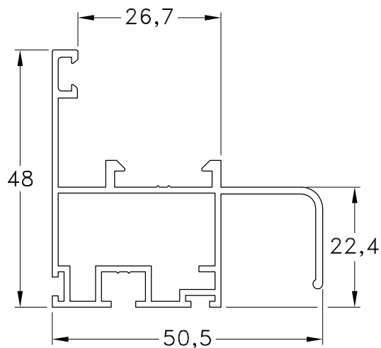
1040506 - Zócalo / Cabezal Peso: 0,69 Kg/m. Largo Std.: 6.030 mm.
