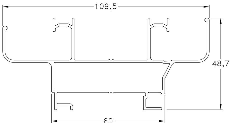
1060697 - Marco Perimetral Peso: 1,20 Kg/m. Largo Std.: 6.030 mm.
