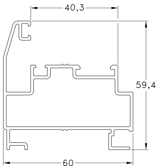
1060894 - Marco Coplanar Peso: 1,02 Kg/m. Largo Std.: 6.150 mm.
