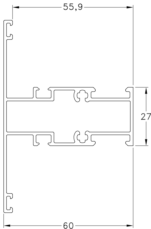
1060780 - Travesaño Peso: 1,11 Kg/m. Largo Std.: 6.030 mm.
