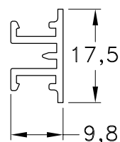
1060540 - Tapa Soporte Paño Fijo Peso: 0,15 Kg/m. Largo Std.: 6.030 mm.
