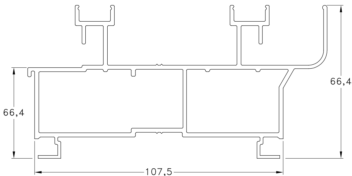
1060601 - Marco Peso: 2,35 Kg/m. Largo Std.: 6.030 mm.
