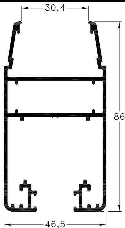
1060555 - Hoja Perimetral Peso: 1,43 Kg/m. Largo Std.: 6.030 mm.
