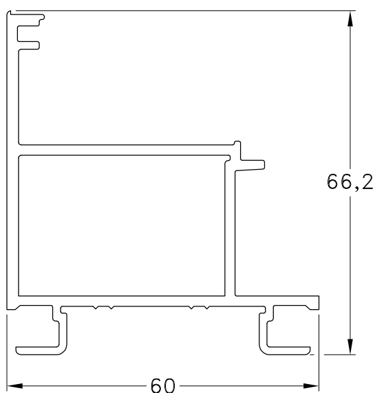
1060860 - Marco Paño Fijo Peso: 1,19 Kg/m. Largo Std.: 6.030 mm.
