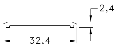
1060565 - Tapa Puerta Vaivén Peso: 0,13 Kg/m. Largo Std.: 6.030 mm.
