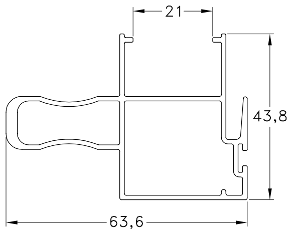
1060817 - Parante Central Ref. D.V.H. Peso: 0,85 Kg/m. Largo Std.: 6.150 mm.
