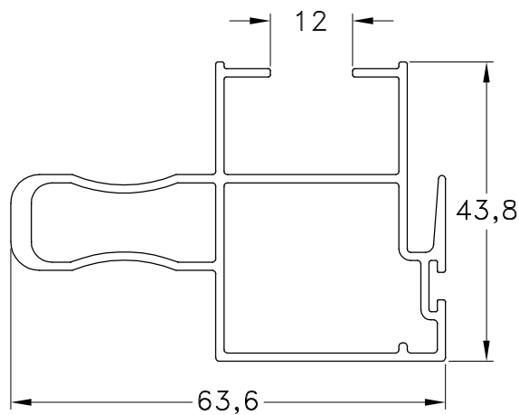
1060834 - Parante Central Ref. V.S. Peso: 0,88 Kg/m. Largo Std.: 6.150 mm.
