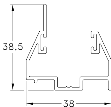
1060577 - Guía Postiza Cortina Peso: 0,49 Kg/m. Largo Std.: 6.150 mm.
