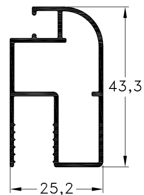
1060108 - Hoja Mosquitero Peso: 0,47 Kg/m. Largo Std.: 6.030 mm.
