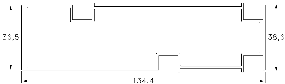
1060855 - Acople Recto Reforzado Peso: 1,59 Kg/m. Largo Std.: 6.030 mm.
