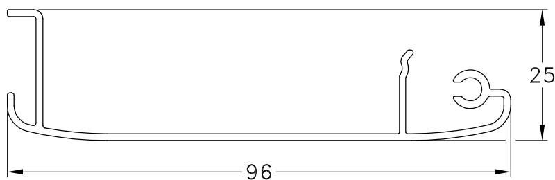
1060683 - Tapacinta Peso: 0,60 Kg/m. Largo Std.: 6.150 mm.
