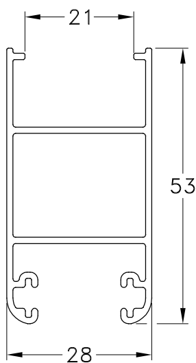
1060819 - Parante Lateral D.V.H. Peso: 0,61 Kg/m. Largo Std.: 6.150 mm.
