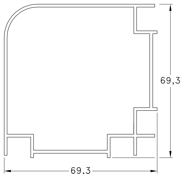
1060564 - Columna Curva a 90°
