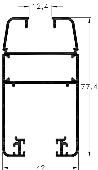
1060881 - Hoja Perimetral V.S. Peso: 1,19 Kg/m. Largo Std.: 6.030 mm.
