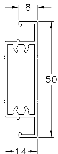
1060190 - Travesaño Mosquitero Peso: 0,45 Kg/m. Largo Std.: 6.030 mm.
