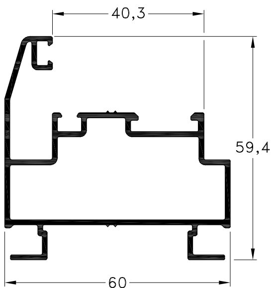
1060896 - Marco Coplanar Peso: 1,03 Kg/m. Largo Std.: 6.150 mm.
