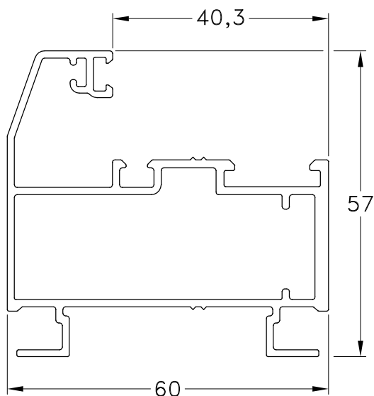
1060890 - Marco C-16 Peso: 1,12 Kg/m. Largo Std.: 6.150 mm.
