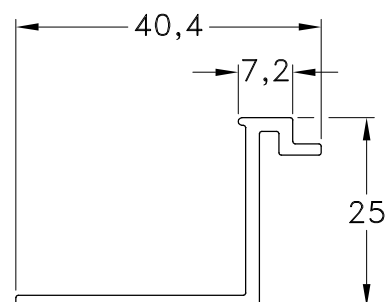
1060611 - Contravidrio de 7,2 mm. Peso: 0,30 Kg/m. Largo Std.: 6.030 mm.
