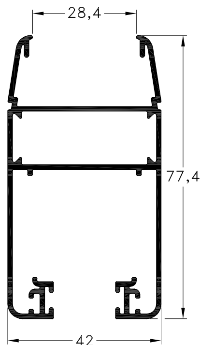
1060882 - Hoja Perimetral D.V.H. Peso: 1,14 Kg/m. Largo Std.: 6.030 mm.
