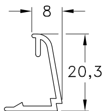
1060526 - Contravidrio Peso: 0,15 Kg/m. Largo Std.: 6.030 mm.
