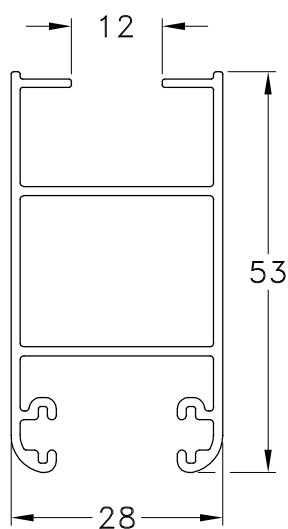
1060823 - Parante Lateral V.S. Peso: 0,64 Kg/m. Largo Std.: 6.150 mm.
