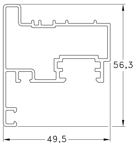
1060825 - Inversor Peso: 0,84 Kg/m. Largo Std.: 6.150 mm.
