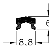
1060561 - Guía Inferior Peso: 0,09 Kg/m. Largo Std.: 6.030 mm.
