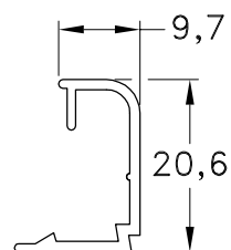
1040510 - Contravidrio D.V.H. Peso: 0,15 Kg/m. Largo Std.: 6.030 mm.
