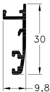
1060884 - Contramarco Peso: 0,20 Kg/m. Largo Std.: 6.150 mm.
