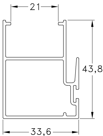
1060816 - Parante Central D.V.H. Peso: 0,57 Kg/m. Largo Std.: 6.150 mm.
