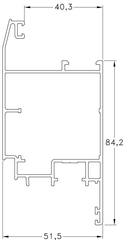
1060889 - Hoja C-16 Peso: 1,30 Kg/m. Largo Std.: 6.150 mm.
