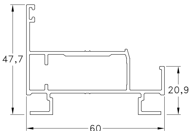
1060883 - Hoja V.R., B. y O.B. Peso: 0,90 Kg/m. Largo Std.: 6.150 mm.
