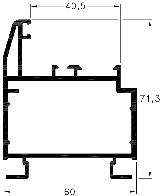
1060541 - Marco Peso: 1,57 Kg/m. Largo Std.: 6.150 mm.
