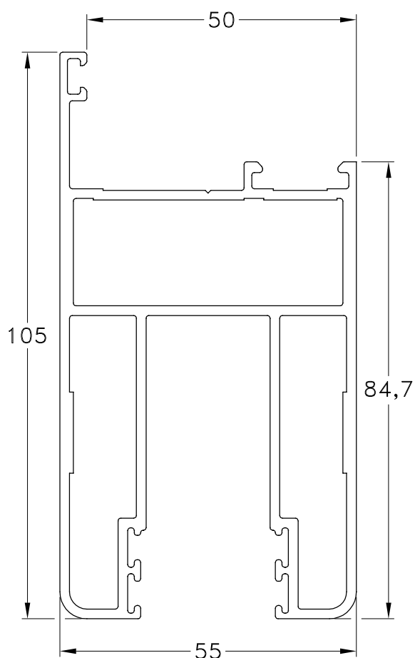
1060602 - Hoja Peso: 2,33 Kg/m. Largo Std.: 6.030 mm.
