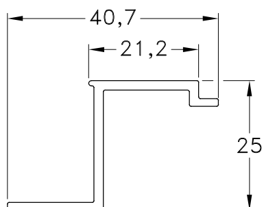
1060612 - Contravidrio de 21,2 mm. Peso: 0,31 Kg/m. Largo Std.: 6.030 mm.
