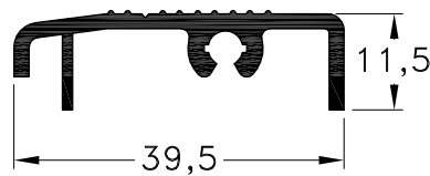
1060726 - Umbral Transitable Peso: 0,39 Kg/m. Largo Std.: 6.030 mm.
