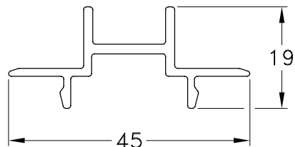
1060607 - Encuentro de Cuatro Hojas Peso: 0,34 Kg/m. Largo Std.: 6.030 mm.
