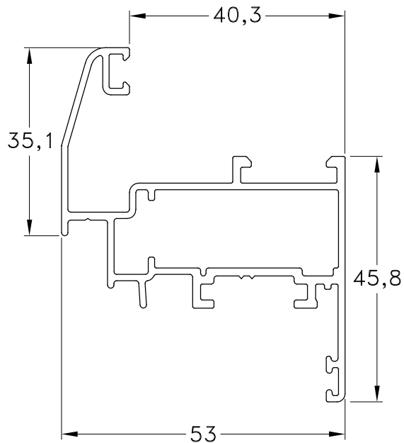
1060883 - Hoja V.R., B. y O.B. Peso: 0,90 Kg/m. Largo Std.: 6.150 mm.
