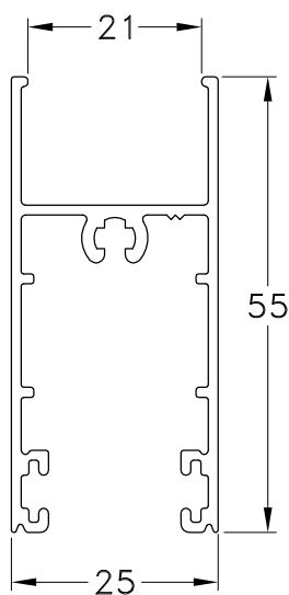
1060815 - Cabezal / Zócalo D.V.H. Peso: 0,59 Kg/m. Largo Std.: 6.030 mm.
