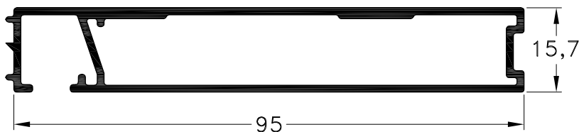
1060875 - Premarco de 95 mm. Peso: 0,88 Kg/m. Largo Std.: 6.150 mm.
