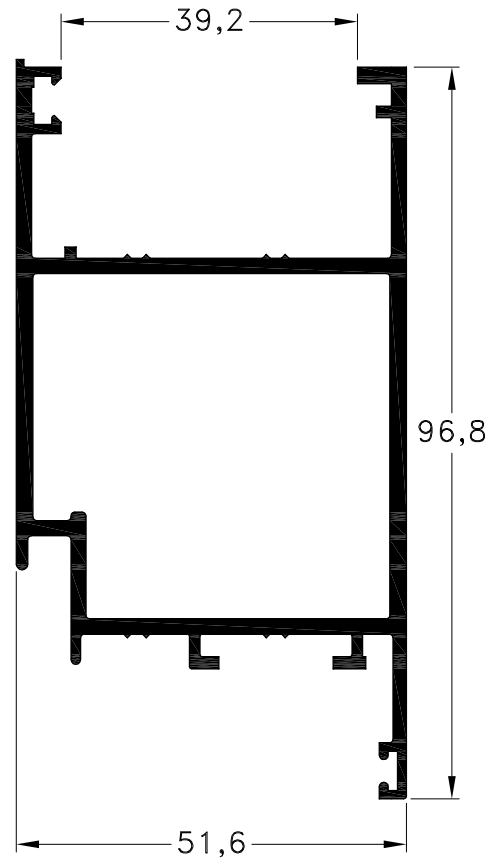
1060547 - Cabezal y Parante de Hoja Peso: 1,66 Kg/m. Largo Std.: 6.150 mm.
