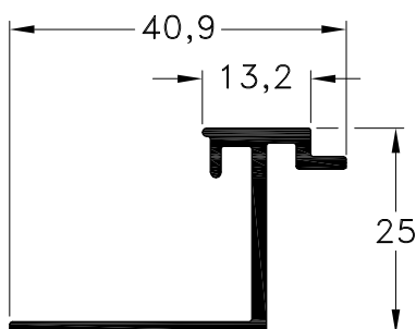
1060546 - Contravidrio de 13,2 mm. Peso: 0,35 Kg/m. Largo Std.: 6.030 mm.
