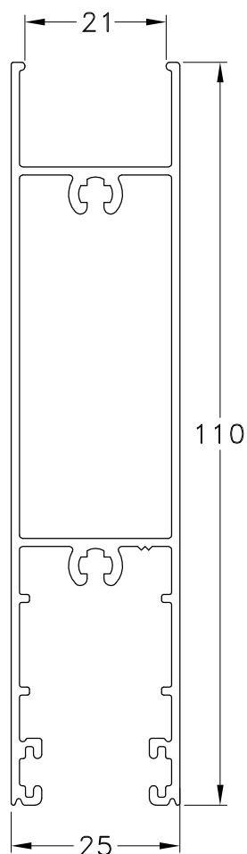
1060818 - Zócalo Alto D.V.H. Peso: 1,08 Kg/m. Largo Std.: 6.030 mm.
