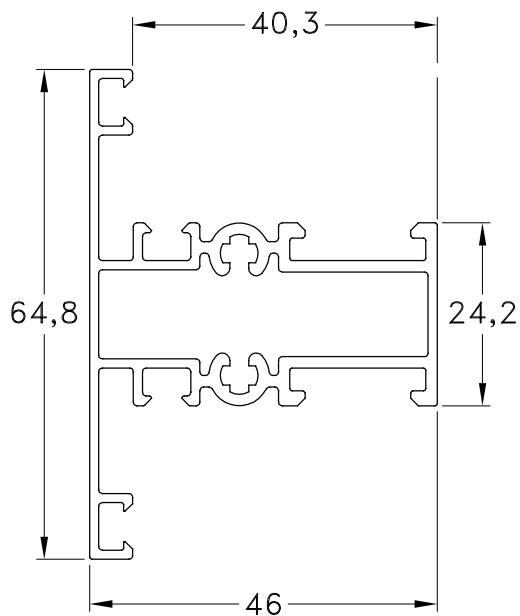
1060835 - Travesaño Angosto Peso: 0,94 Kg/m. Largo Std.: 6.030 mm.
