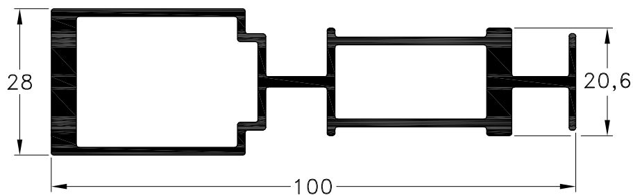
1060850 - Acople Recto Reforzado Peso: 1,55 Kg/m. Largo Std.: 6.030 mm.
