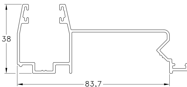
1060578 - Guía Cortina Común Peso: 0,81 Kg/m. Largo Std.: 6.150 mm.
