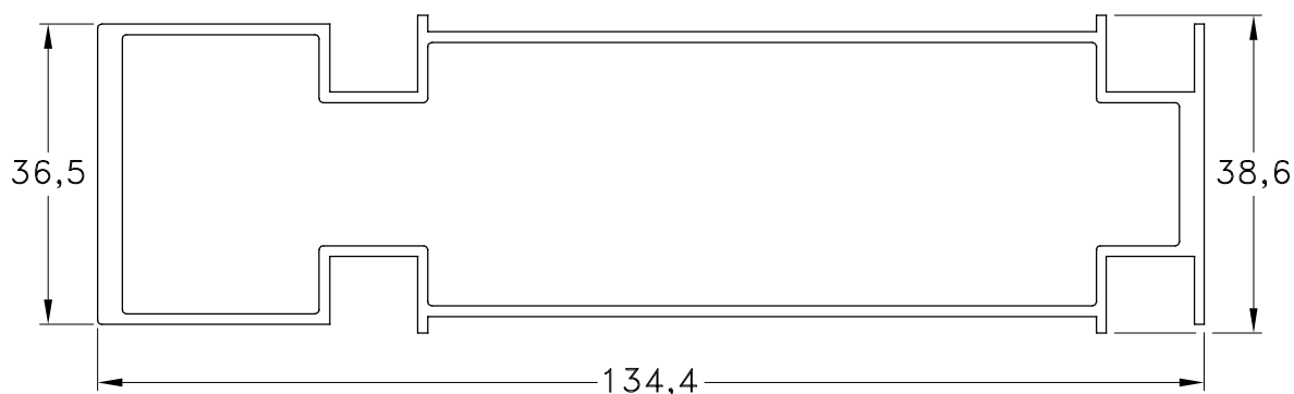
1060854 - Acople Recto Reforzado Peso: 1,60 Kg/m. Largo Std.: 6.030 mm.
