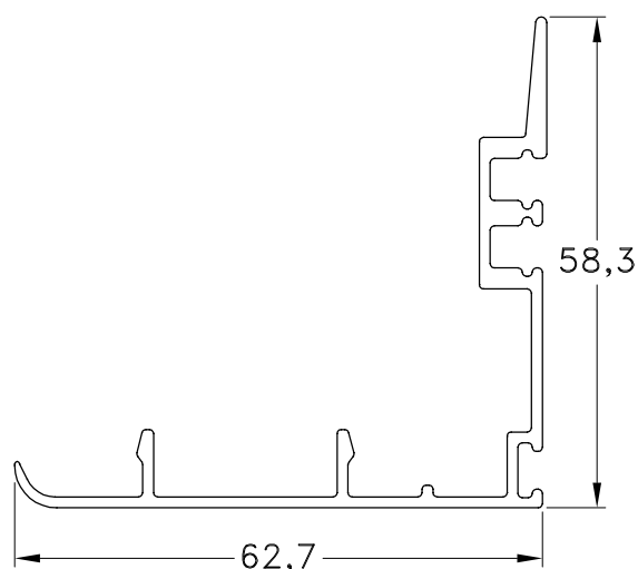
1060609 - Encuentro Peso: 0,66 Kg/m. Largo Std.: 6.030 mm.
