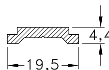
9469 - Pletina de Poliamida Largo Std.: 6.150 mm.
