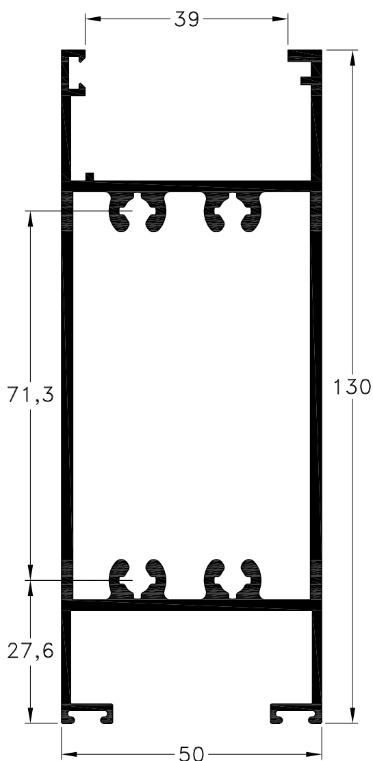
1060542 - Zócalo Reforzado Peso: 2,55 Kg/m. Largo Std.: 6.030 mm.
