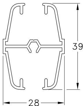
1060747 - Travesaño V.R. Peso: 0,45 Kg/m. Largo Std.: 6.030 mm.
