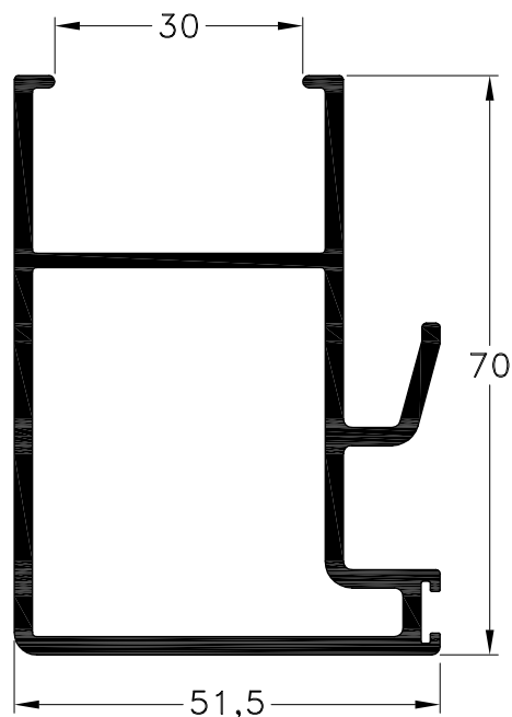
1060169 - Parante Central M-Cinco Peso: 1,48 Kg/m. Largo std.: 6.150 mm.
