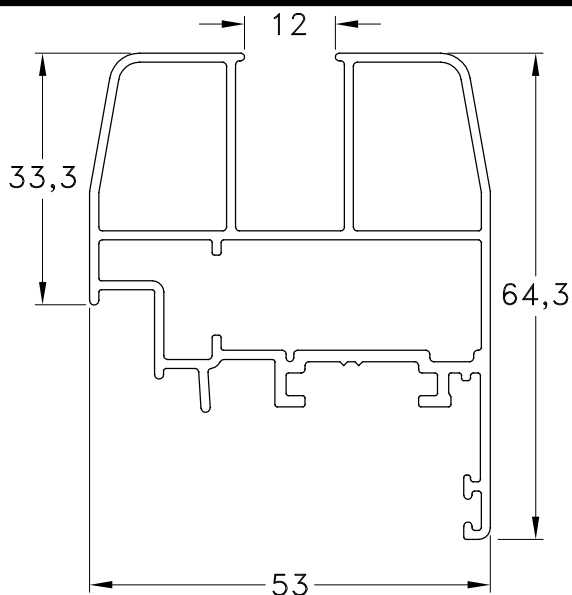
1060827 - Hoja V.S. Peso: 1,09 Kg/m. Largo Std.: 6.150 mm.
