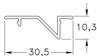
1040509 - Tapa Compensador Peso: 0,14 Kg/m. Largo Std.: 6.030 mm.
