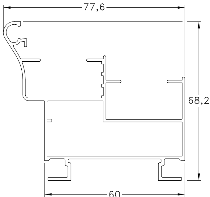
1060512 - Marco Peso: 1,05 Kg/m. Largo Std.: 6.030 mm.
